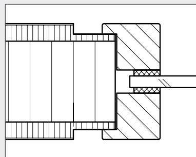
Detail: Classique light mit Verglasung und flächenbündiger Glasleiste
